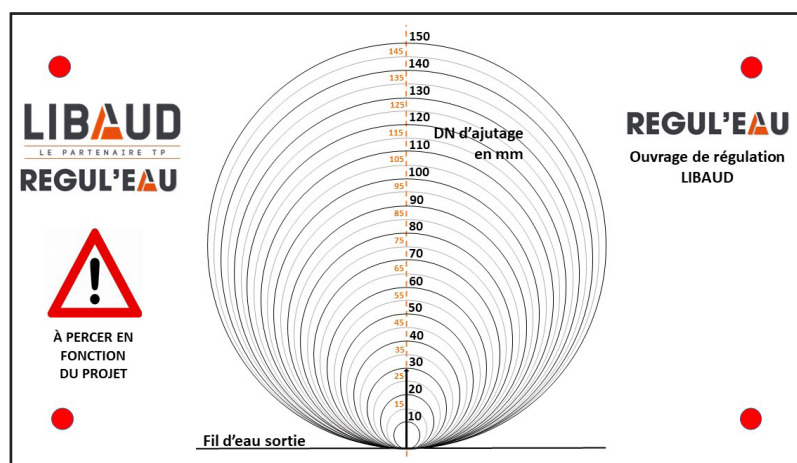
ECHELLE D'AJUTAGE CALBRÉE
