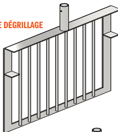
3 - PELLE DE REGULATION AVAL
