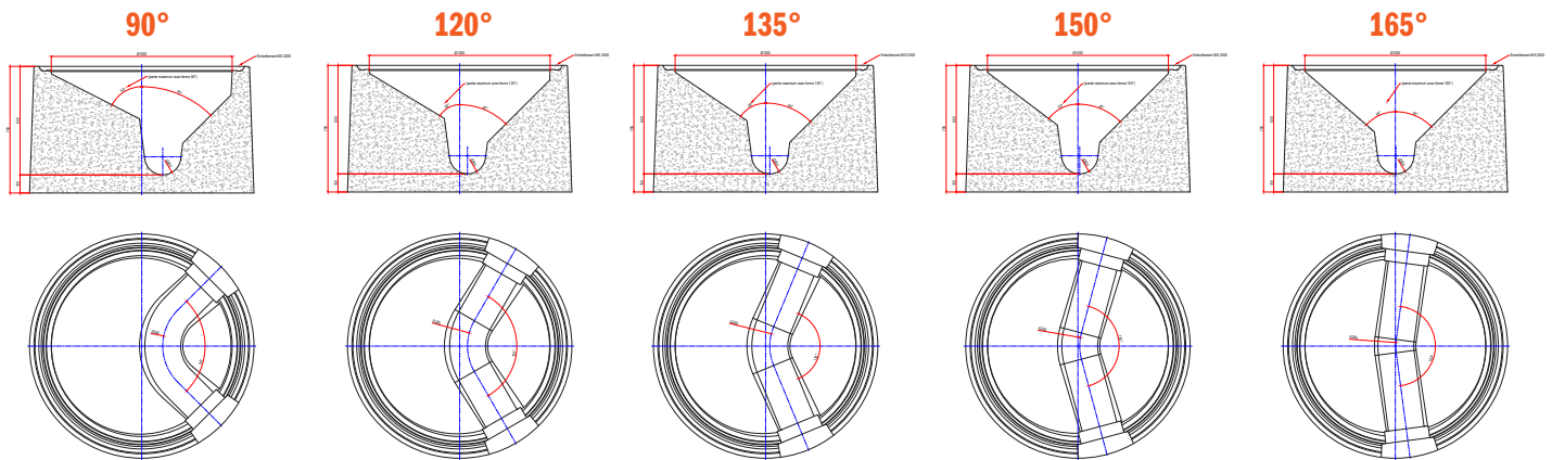
Cunette réversible sans pente
