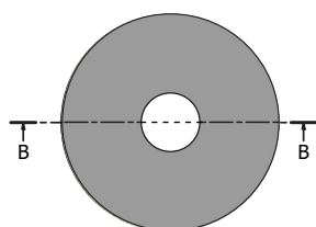
DALLE DE COUVERTURE DN 600 TROU CENTRÉ
