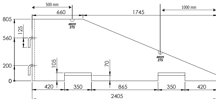
PLAN SIFFLET CROCHET
