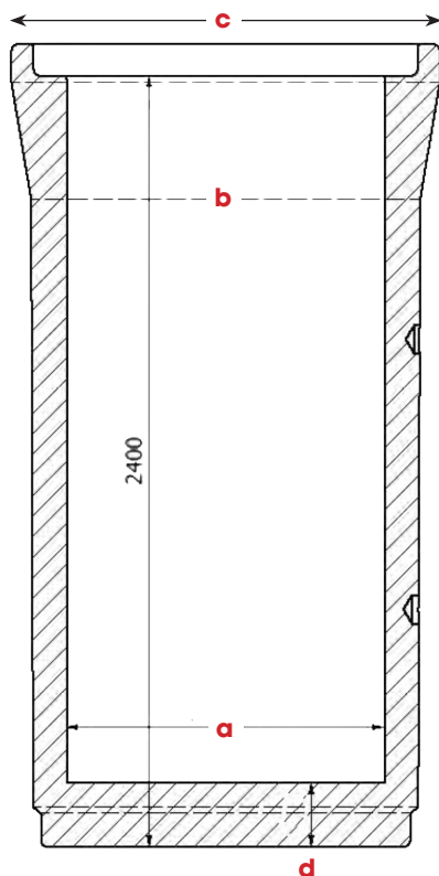
Tuyau obturé mâle
