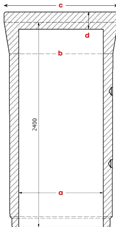
Tuyau obturé femelle
