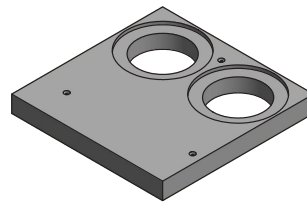
DALLE RÉDUCTRICE 180 X 180 DOUBLE ACCÈS TH DN600 - VOIRIE
